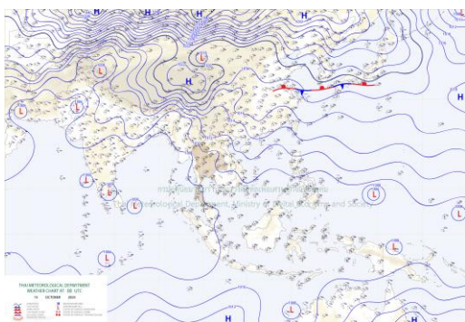
แผนที่อากาศผิวพื้น วันที่ 15 ตุลาคม 2568 เวลา 07:00
