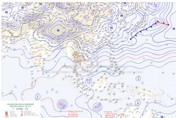
แผนที่อากาศผิวพื้น วันที่ 18 ธันวาคม 2568 เวลา 07:00 น.
