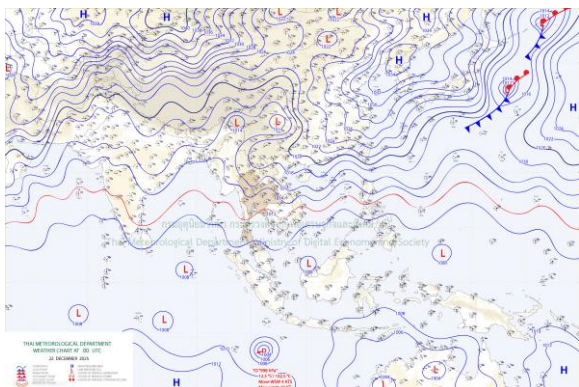
แผนที่อากาศผิวพื้น วันที่ 22 ธันวาคม 2568 เวลา 07:00 น.
