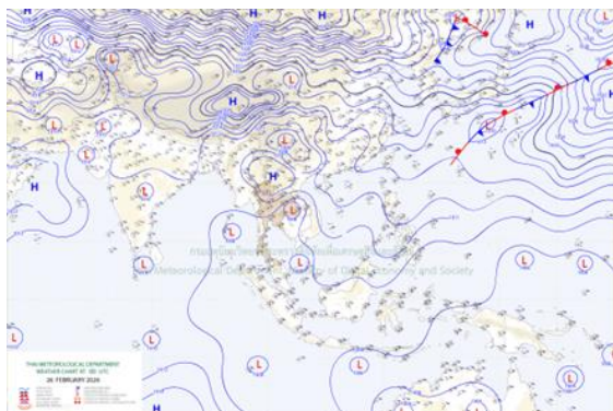
แผนที่อากาศผิวพื้น วันที่ 26 กุมภาพันธ์ 2569 เวลา 07:00 น.
